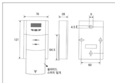
Fig 1. Dimension
