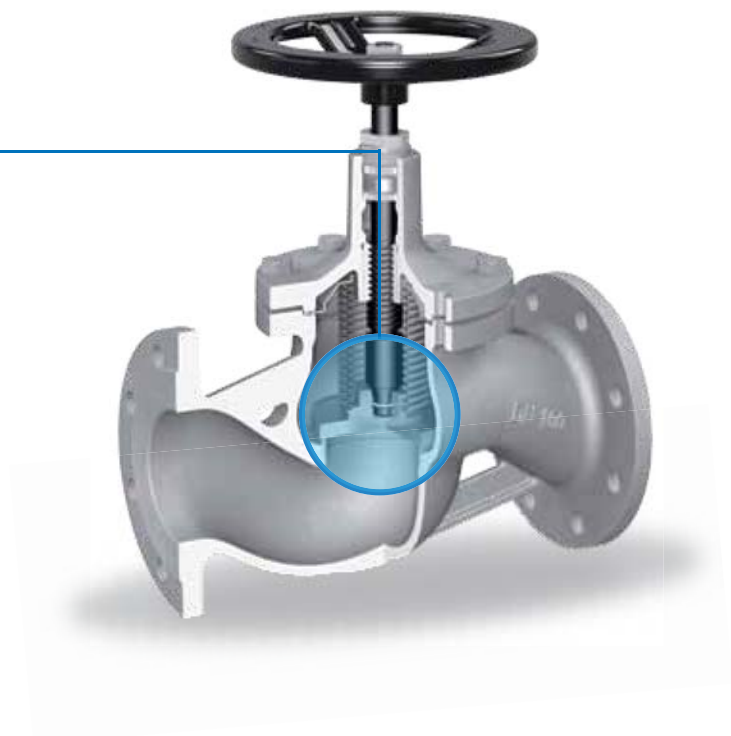
Otturatore a tenuta morbida di PTFE intercambiabile Soft sealing interchangeable PTFE disc
